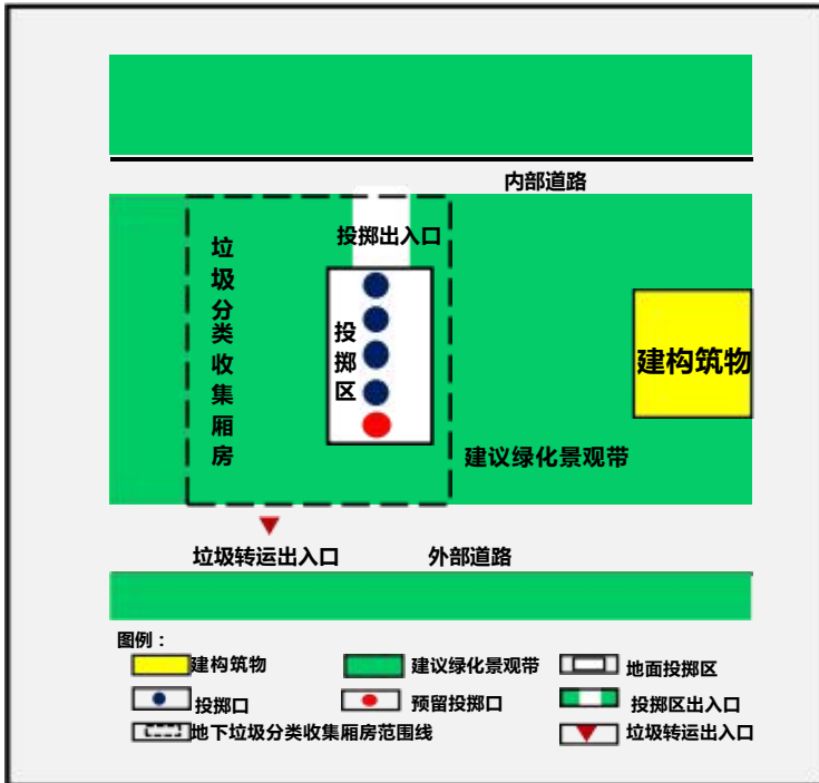
图 6.2 垃圾分类收集厢房地面预留投掷口布局示意
