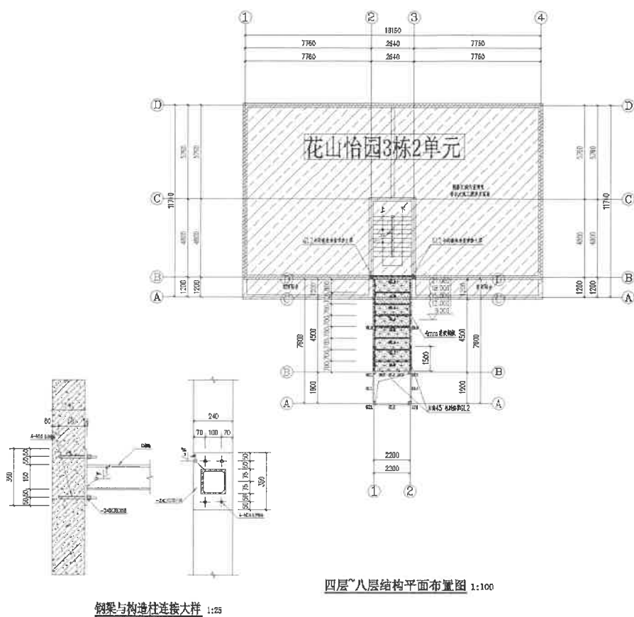
图 2-1 新增电梯标准层结构平面布置
