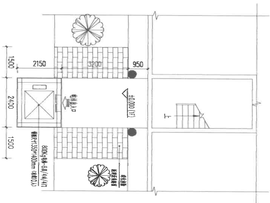
首层原始+新增电梯平面设计图 1:100
