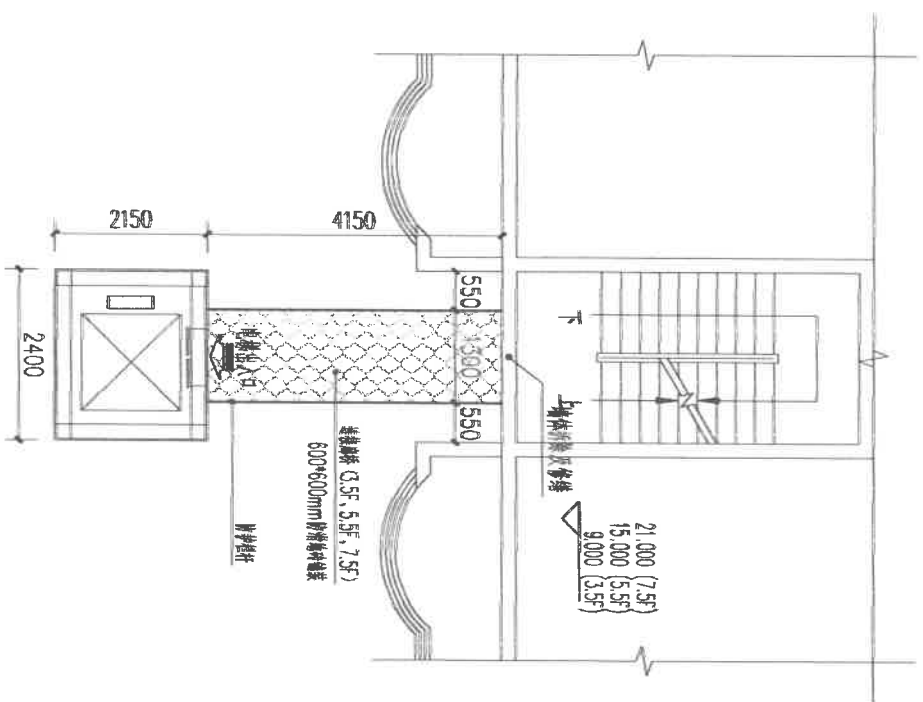
标准层原始+新增电梯平面示意图 1:100
