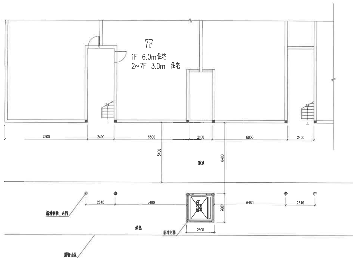
南川区世纪广场小区3栋6.7单元增设电梯一层示意图
