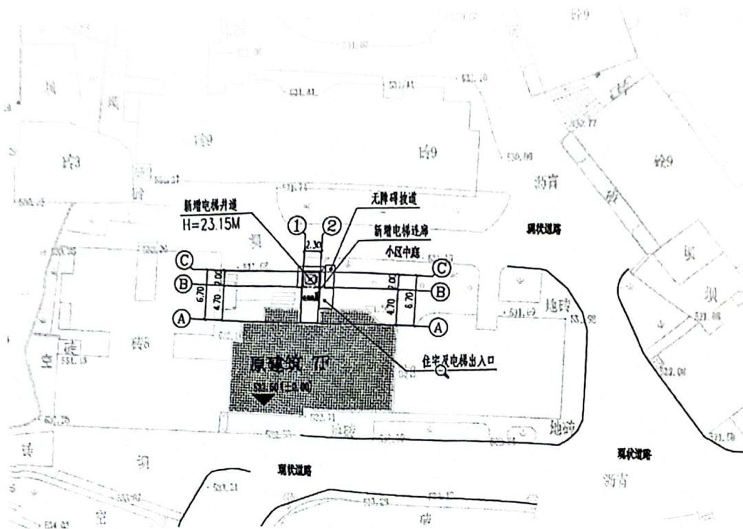
图二：加装室外电梯总平面布置图
