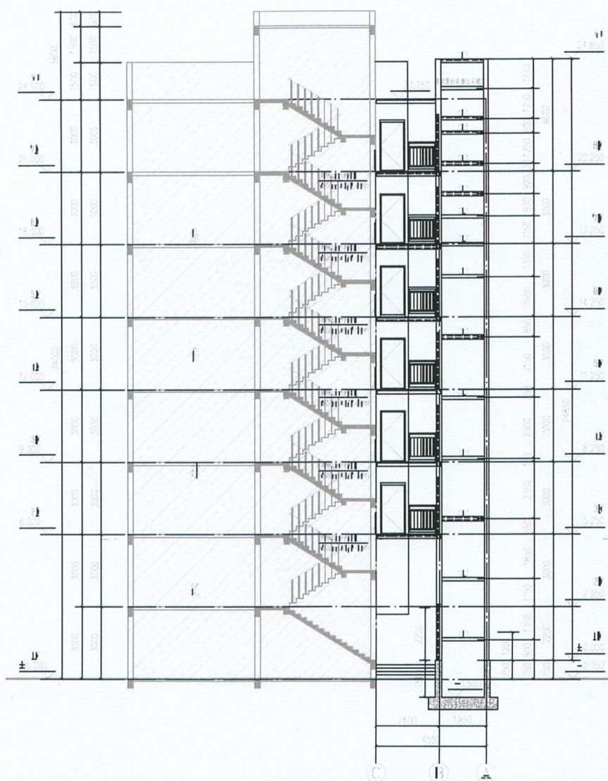
图 2-2 新增电梯标准层结构立面布置
