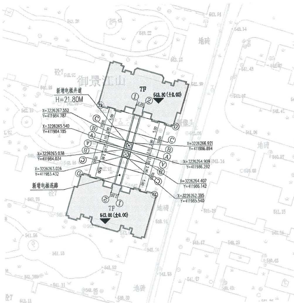
图二：加装室外电梯总平面布置图
