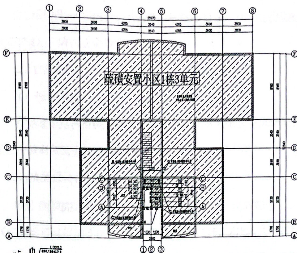
图 2-1 新增电梯标准层结构平面布置
