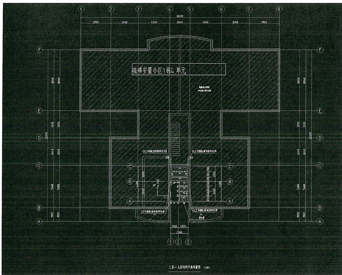
图 2-1 新增电梯标准层结构平面布置
