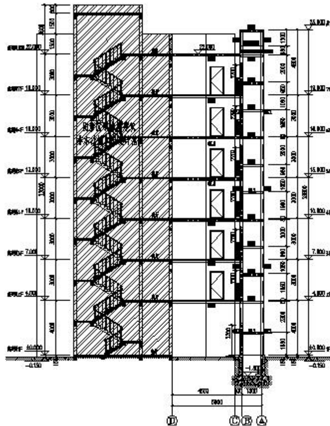
图 2-2 新增电梯标准层结构立面布置
