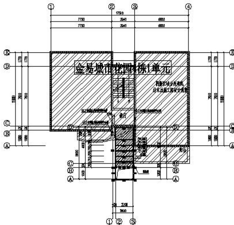
图 2-1 新增电梯标准层结构平面布置
