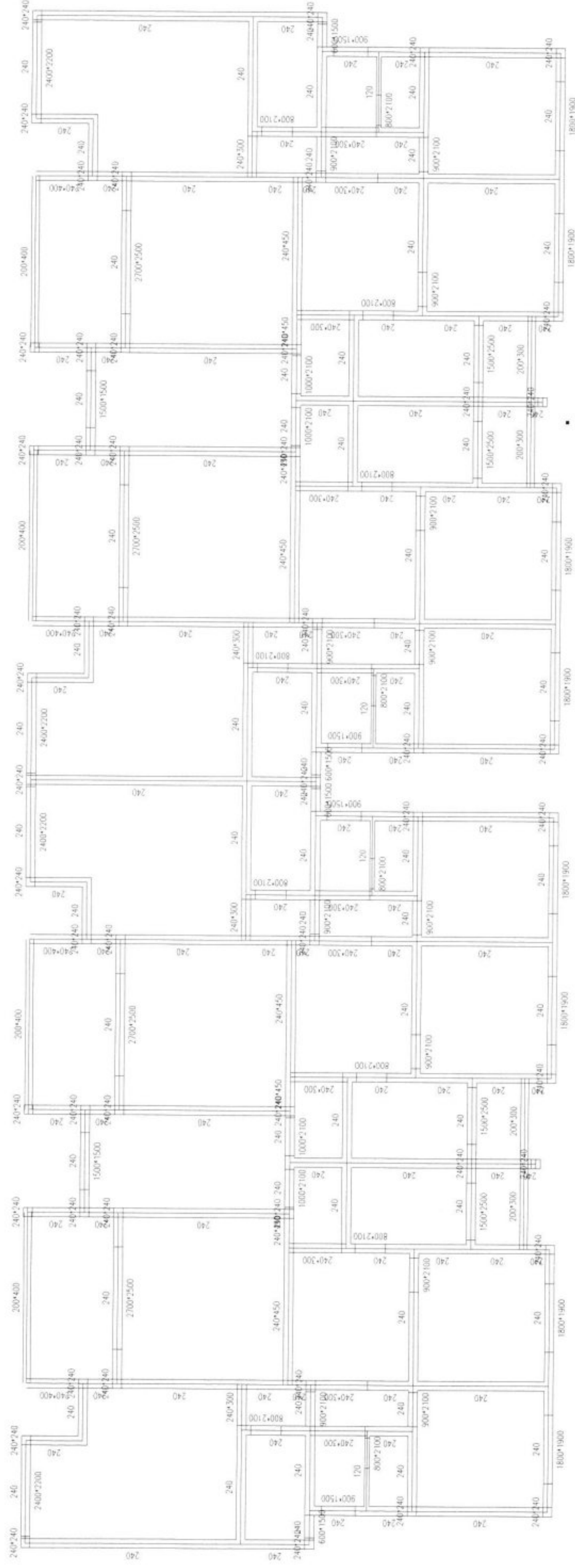
图 4-3 二~六层构件编号
