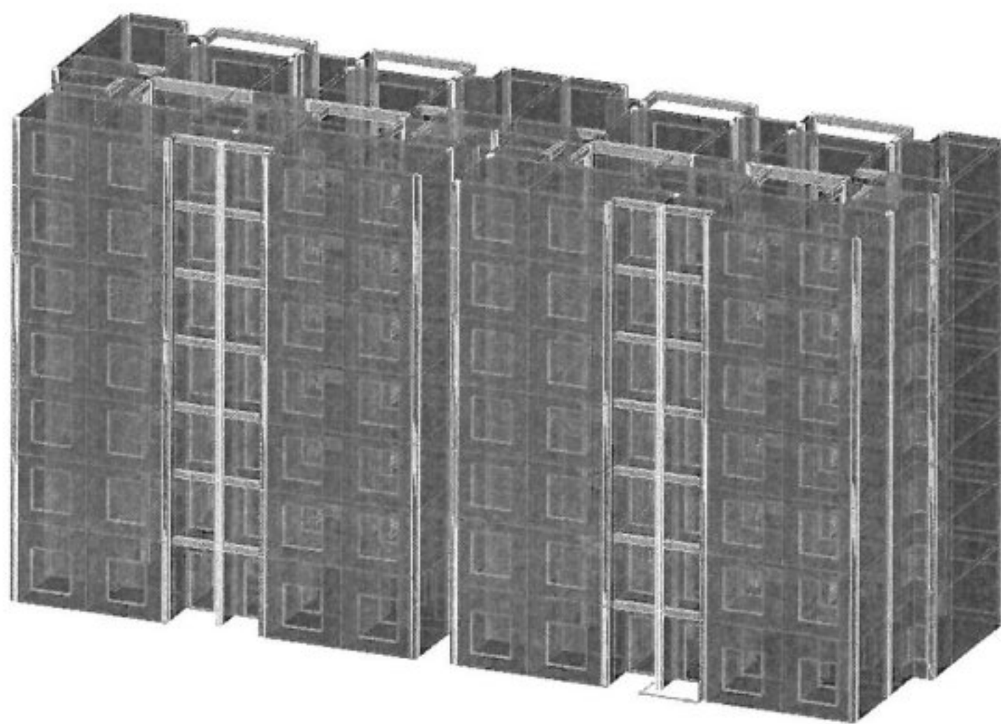
图 6-1 验算模型
