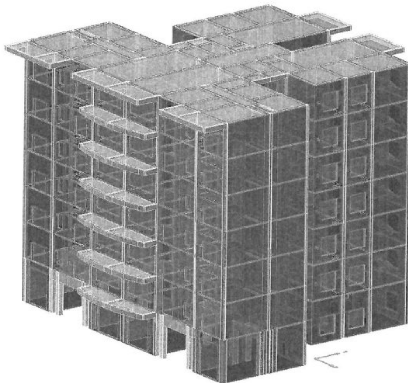
图 6-1 验算模型
