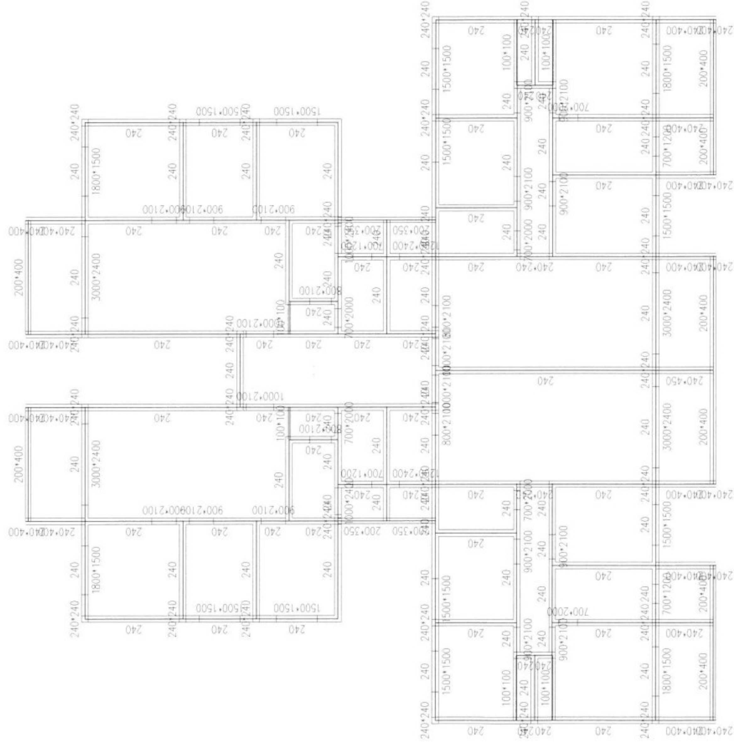
图 4-4 七层构件编号
