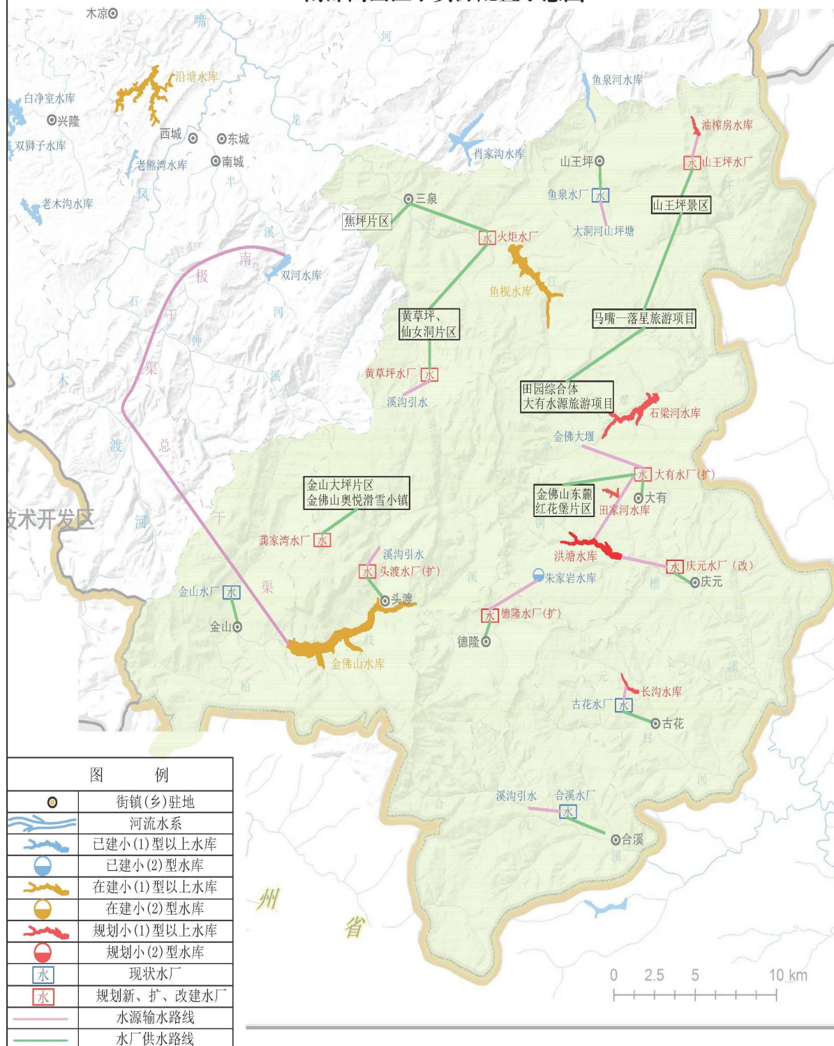
南部高山区水资源配置示意图
